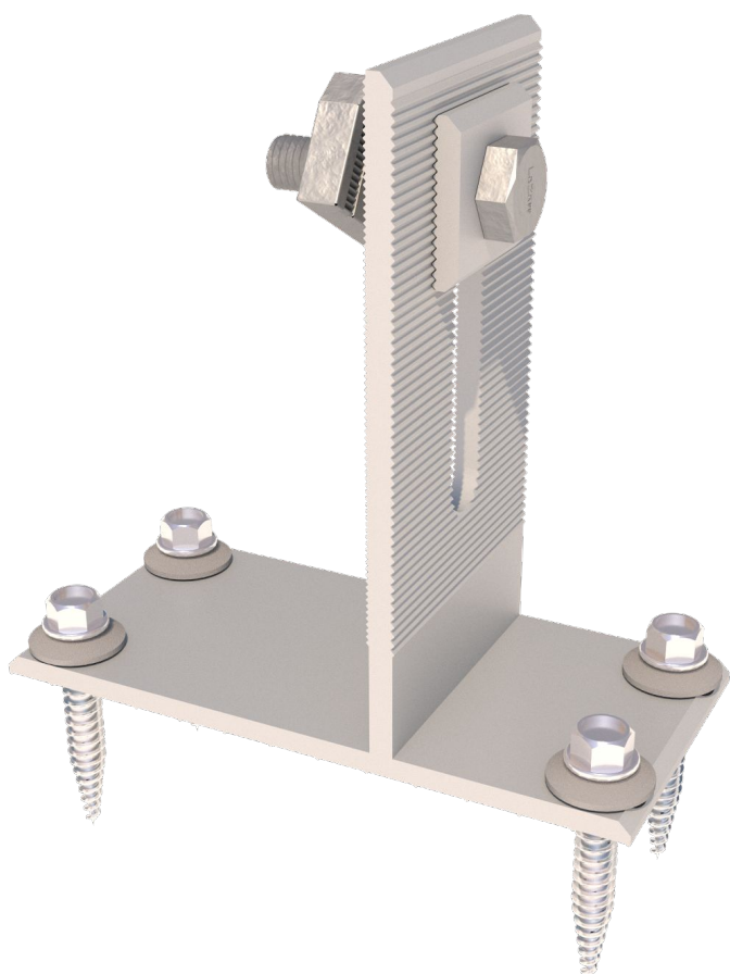
Кронштейн Т-подібний для бітумної черепиці з метизами
